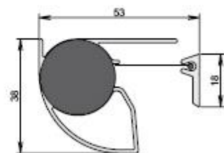
FP400 Dimensions
